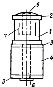
Рис. 21. Пуля Ширинского-Шихматова: 1 — корпус; 2 — ведущие пояски, сжимающиеся при прохождении через чок; 3 — картонные прокладки; 4 — войлочный пыж; 5 — эксцентричная пустота; 6 — свинцовый хвостовик; 7 — надрезы
