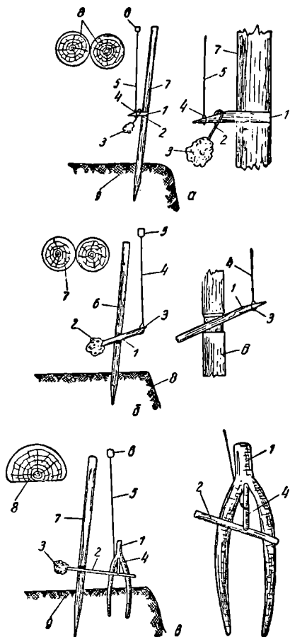
Рис. 13. Спускные механизмы пастей: а) 1 — упорный кольшеш; 2 — кольцо-насторожка, 3 — наживка; 4 — петелька-сторожок; 5 — боевая сямка; 6 — мотырь; 7 — кол коридорчика; 8 — гнет; 9 — земляной холмик; б) 1 — насторожка; 2 — палочка; 3 — петелька-сторожок; 4 — боевая сямка; 5 — мотырь; 6 — кол коридорчика; 7 — гнет; 8 — земляной холмик; в) 1 — развилка-лопатка; 2 — наживная палочка-насторожка; 3 — наживка; 4 — сторожок; 5 — боевая сямка; 6 — мотырь; 7 — кол коридорчика; 8 — гнет; 9 — земляной холмик.
